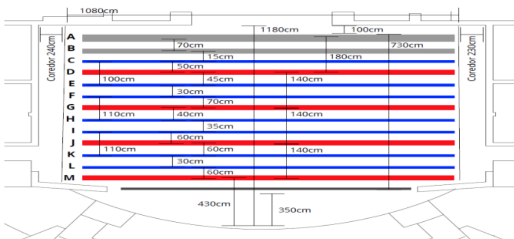
IMAGEM 02 – Medidas de palco
